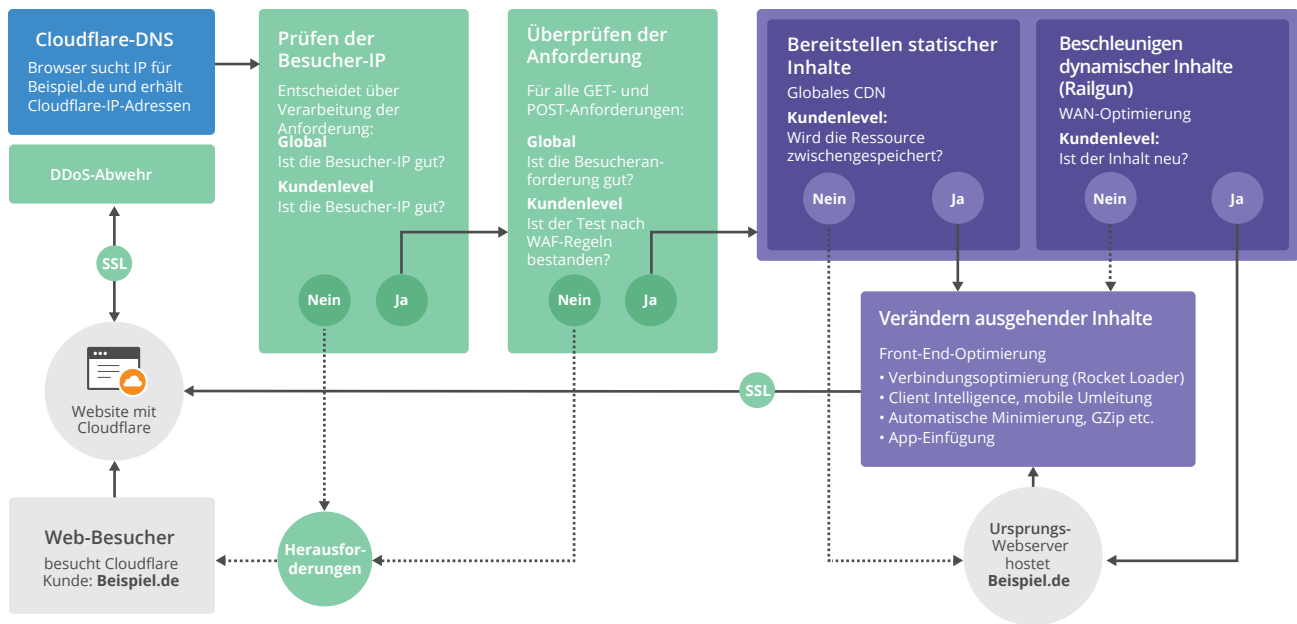
● DNS ● Sicherheit ● Leistung Hinweis: SSL ist optional und wird für jeden Traffic unterstützt. Jeder Knoten im Cloudflare-Netzwerk kann jede Aufgabe ausführen.
